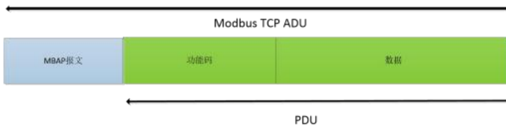
图 34 Modbus TCP 帧
