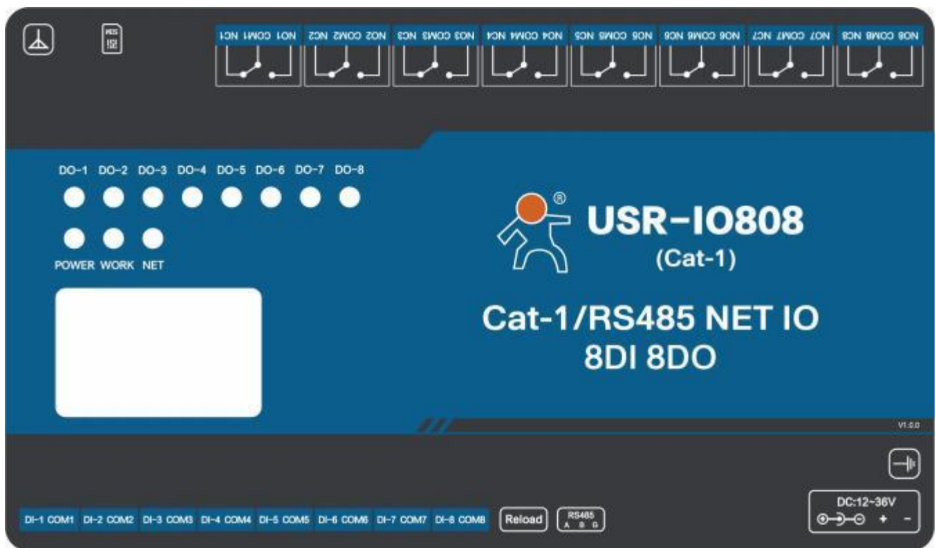
图 13 USR-IO808-CAT1 硬件接口示意图
